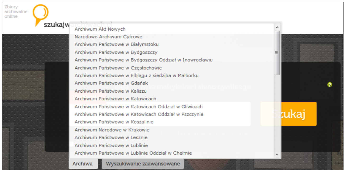
Rys. 8 Wybór archiwum
